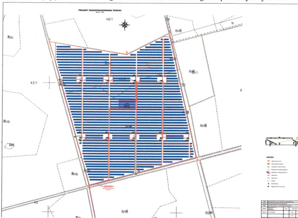
Rozmieszczenie planowanych elementów instalacji zgodnie z planem zawartym w raporcie.
