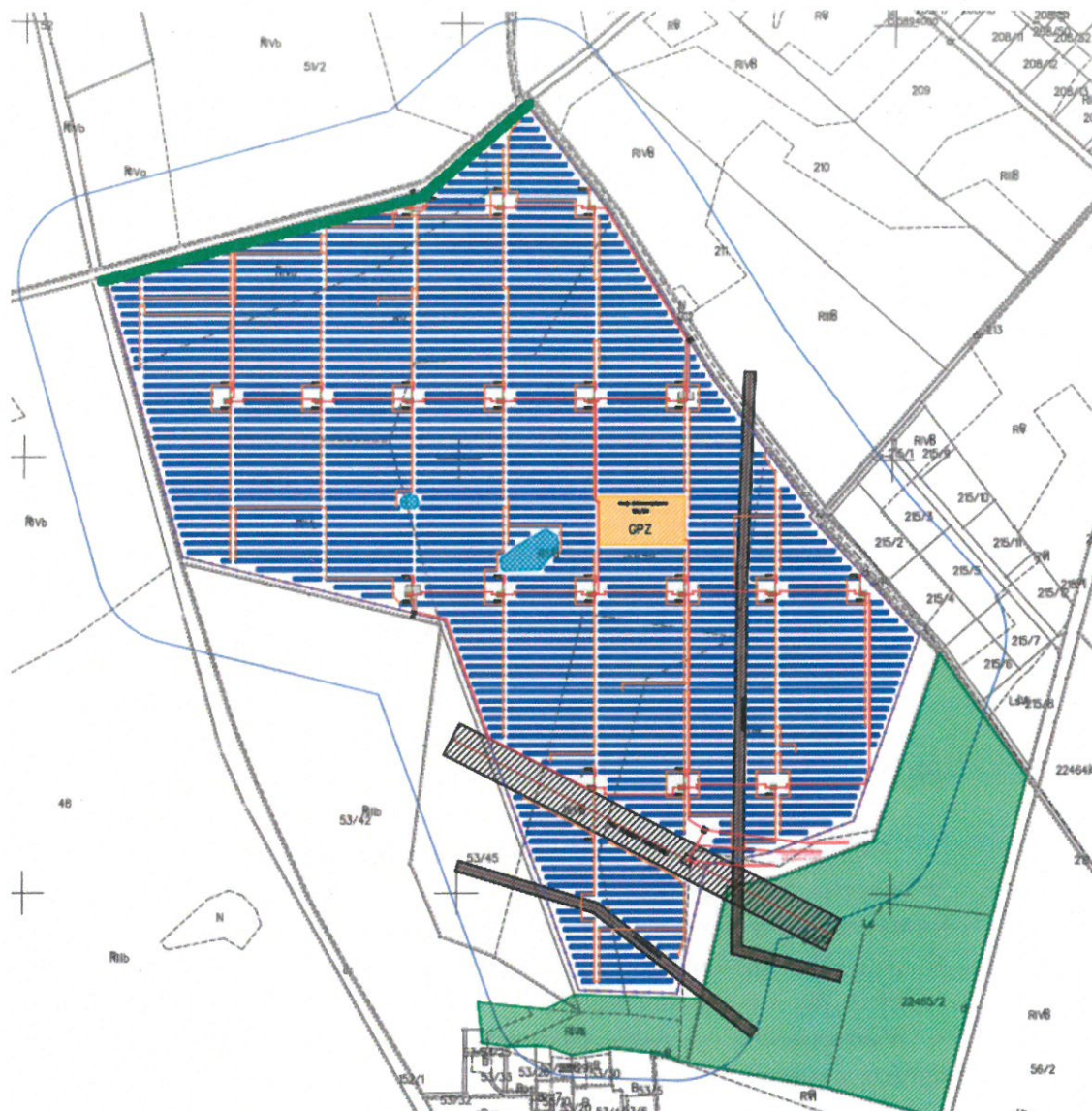
Rysunek 1. Plan nasadzeń zieleni izolacyjnej (zielona pogrubiona linia) zgodny z uzupełnieniem raportu z dnia 30.06.2022 r. (wpływ: 04.07.2022 r.)
