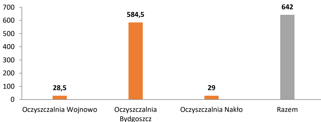
Wykres. Długość wybudowanych i odebranych przyłączy kanalizacyjnych w 2021 r.
