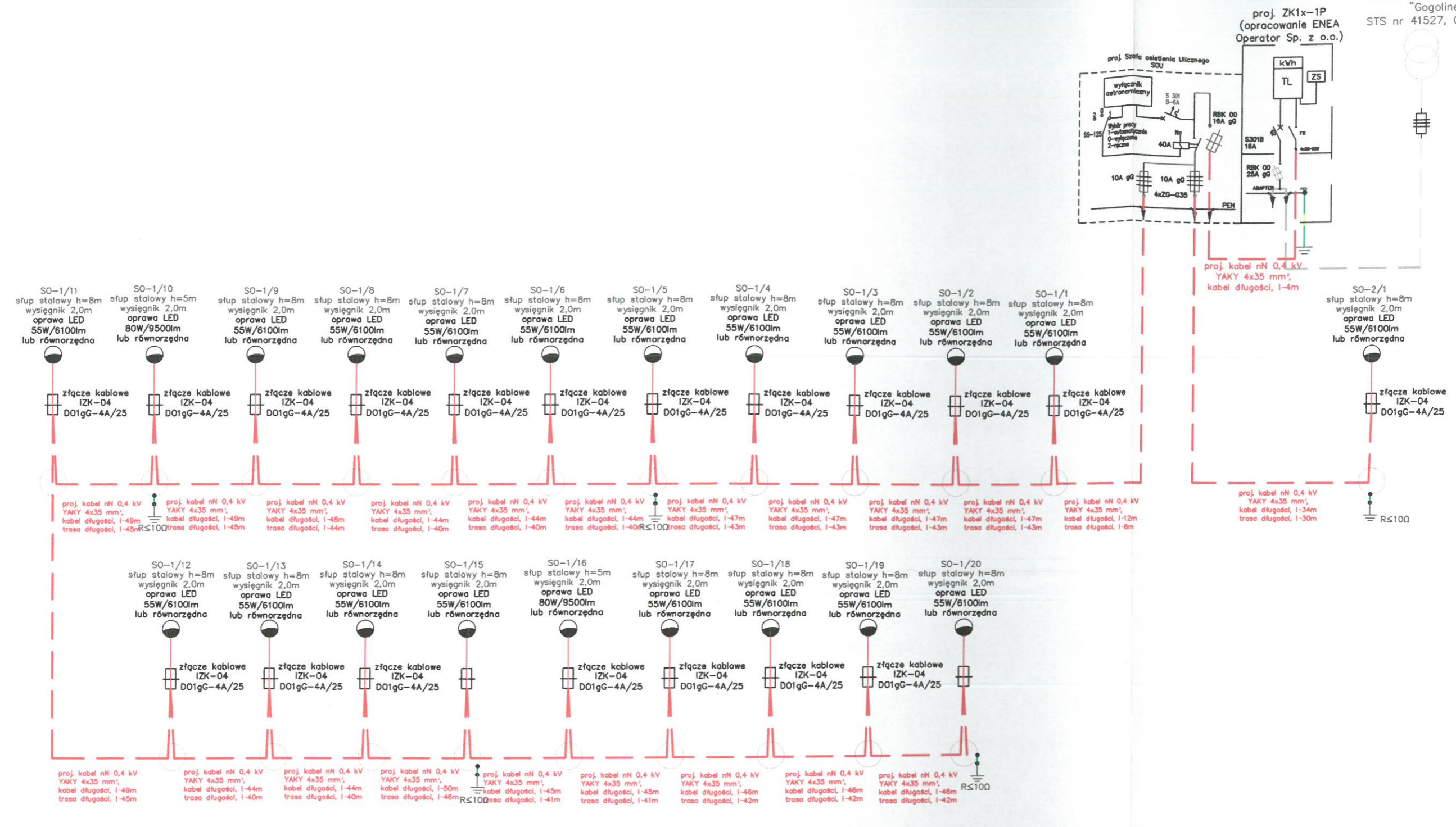
SCHEMAT 1 – KRESKOWY UKŁAD SIECI TN-C
